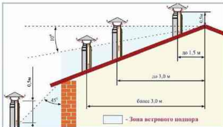
Рис. 7 Высота дымохода.
