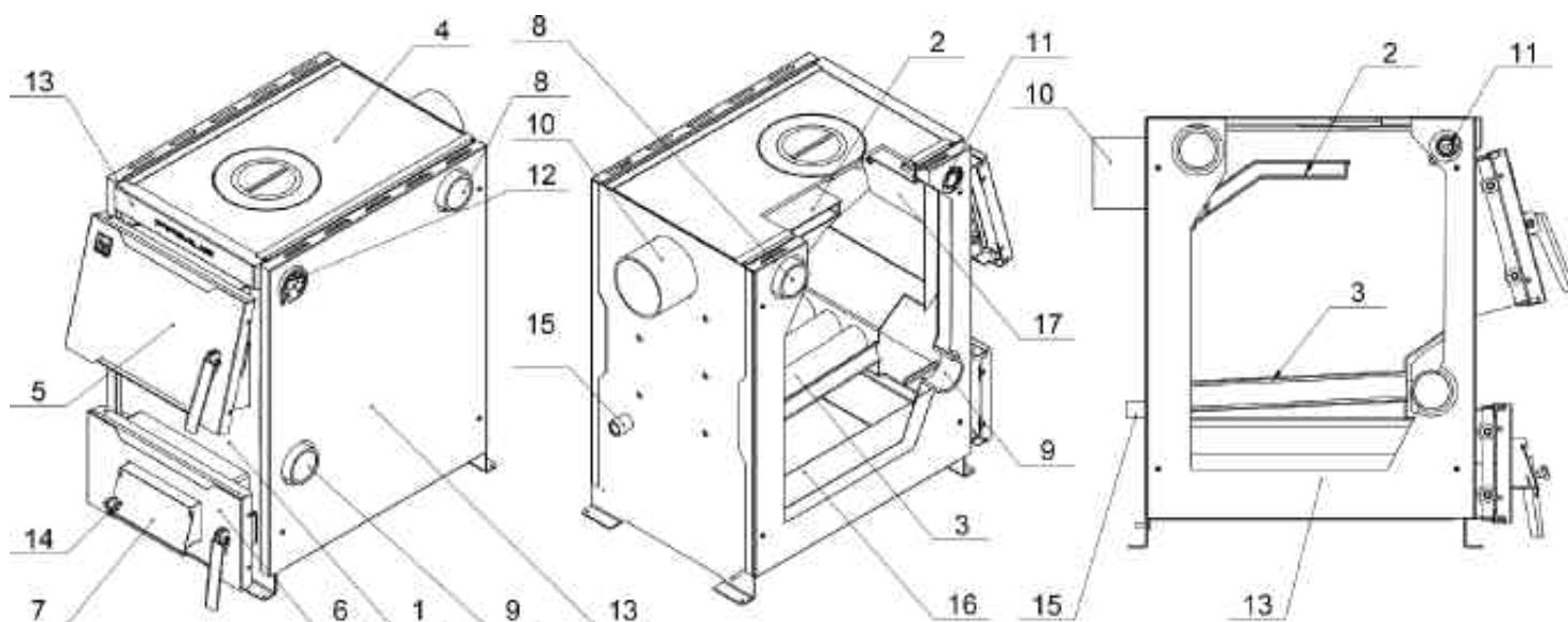
Рис. 1 Устройство котла
